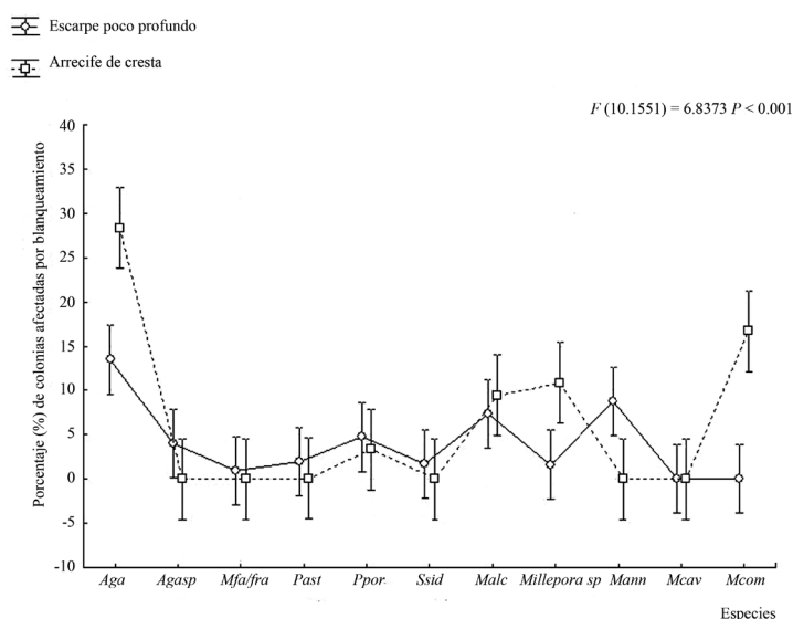
Fig. 2. Porcentaje de blanqueamiento, por especies, en el arrecife de cresta y en el arrecife frontal somero. Leyenda: Agaricia agaricites (Aga), Agaricia sp (Agasp), Montastraea franksi favolata (Mfa/fav), Porites asteroides (Past), Porites porites (Ppor), Siderastrea siderea (Ssid), Millepora alcicornis (Malc), Montastraea annularis (Mann), Montastraea cavernosa (Mcav), Millepora complanata (Mcom)
